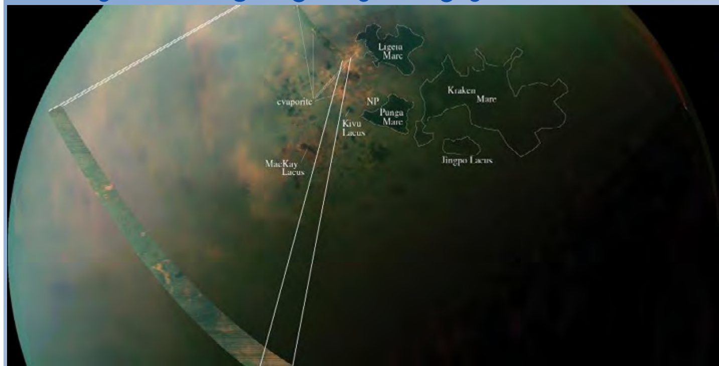
Nowe zdjęcie Tytana - źródło: NASA / Cassini
