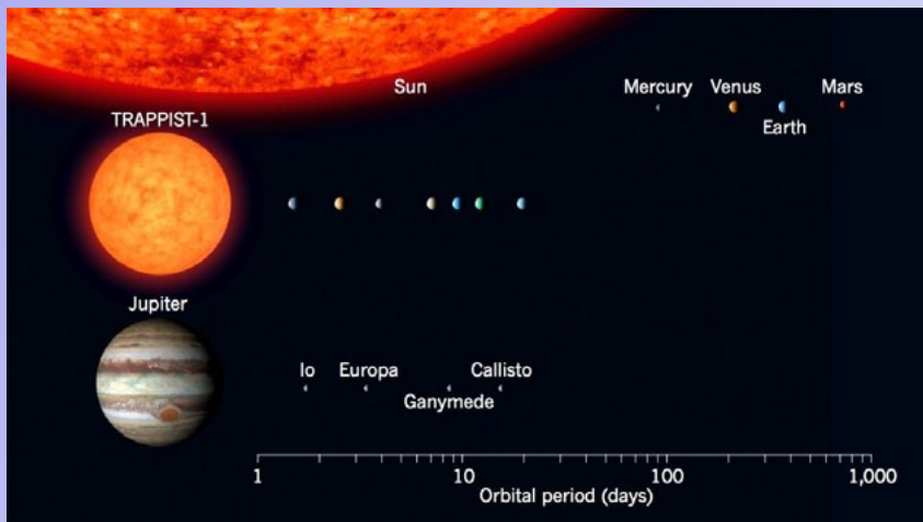
Porównanie układu TRAPPIST-1 do wewnętrznego Układu Słonecznego oraz do księżyców krążących wokół Jowisza / Credits – NASA
